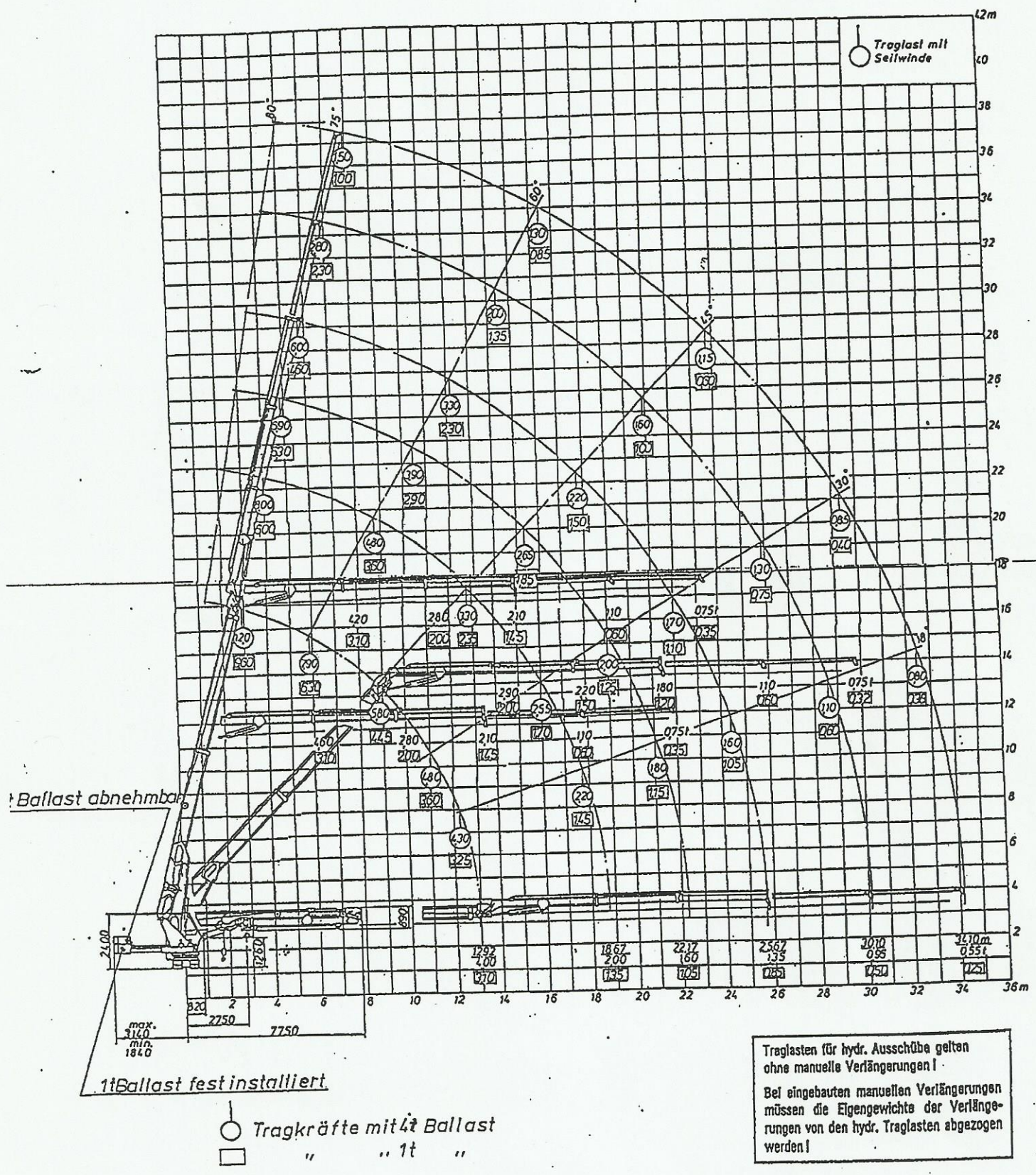
Traglastdiagramm HMK 750 Ta1-a2 load diagram
